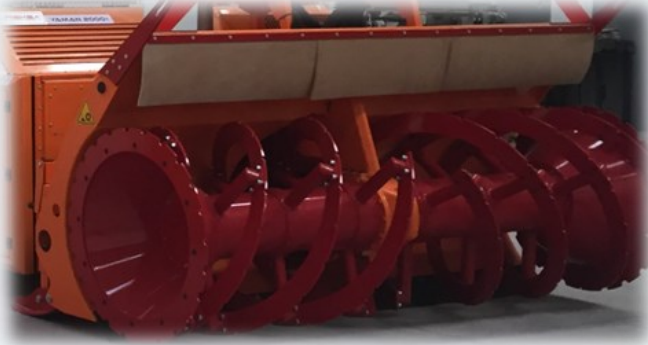
Aşınmaya Dayanıklı Hardox Tambur ve Kesici Bıçakları
