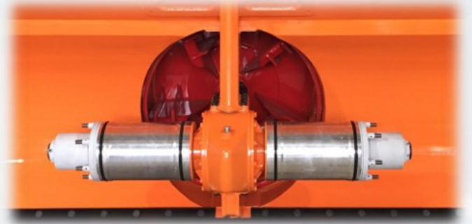
6000 Nm Dayanım Ayarlanabilir Güvenlik Kavramaları
